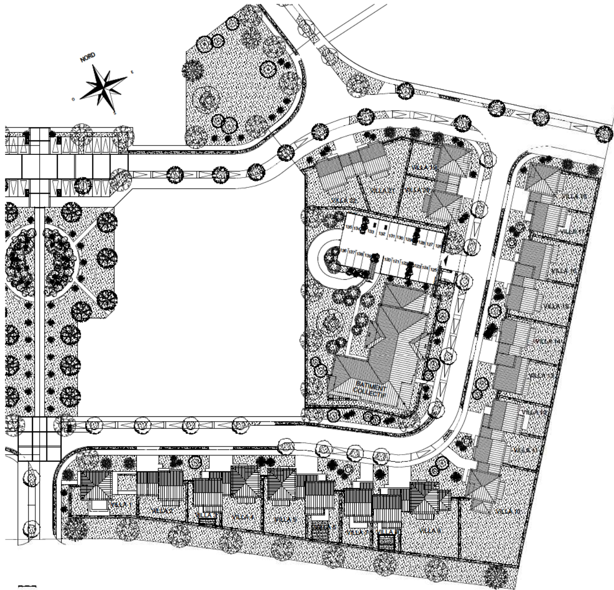
PLAN MASSE
